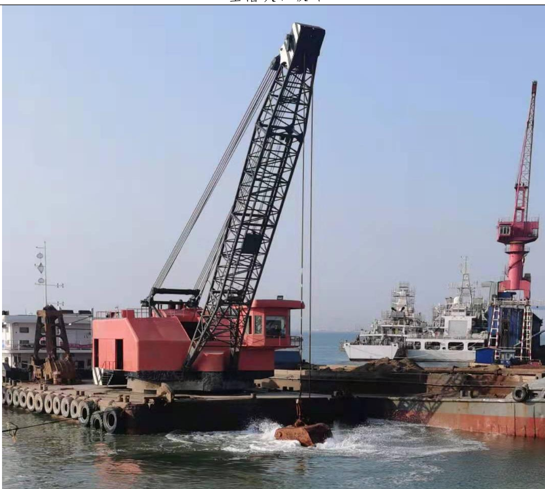
基槽疏浚挖泥
