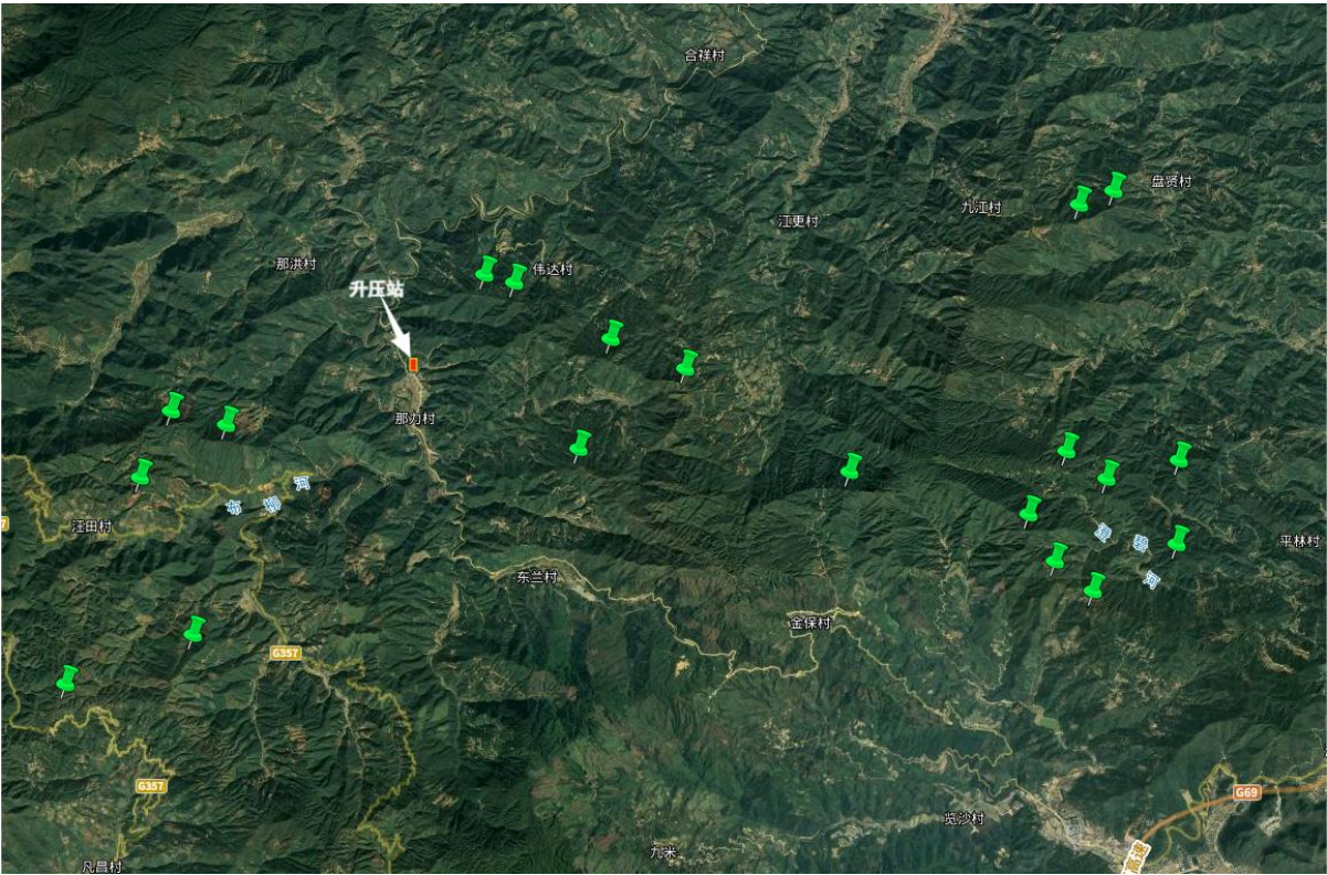
项目风机点位及升压站位置图
